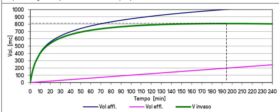
Fig. 14. Sviluppo del volume complessivo in ingresso e in uscita dal sistema e del volume di invaso necessario (differenza tra le due precedenti grandezze) in funzione della durata di precipitazione.
